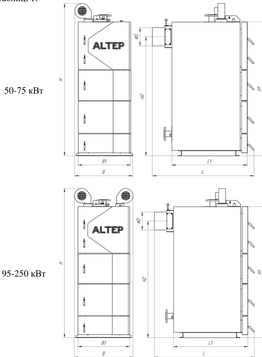
Рисунок 1 – Габаритне креслення котла типу КТ-2Е-N
